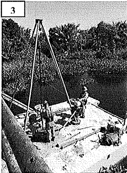
Fotografías 1-4: Ejecución de prueba de penetración estándar con personal especializado.
